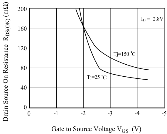
Fig7. R_{DS(ON)} - V_{GS}
