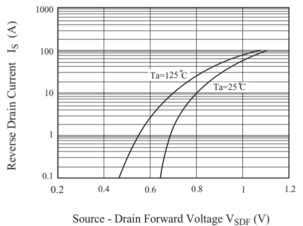
Fig6. I_S - V_{SDF}
