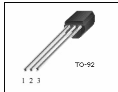
1 - Затвор 2 - Сток 3 - Исток
