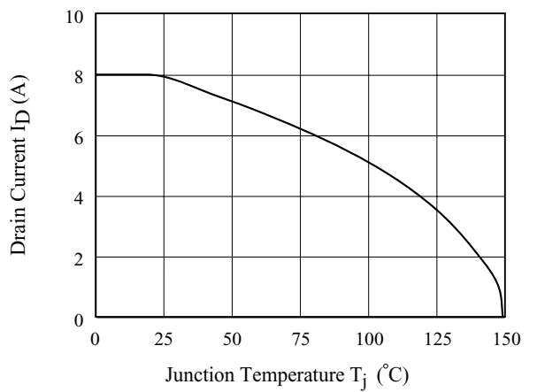
Fig10. I D - T J
