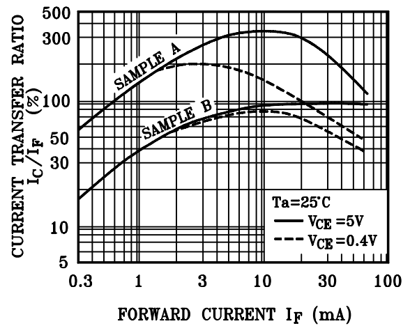
I_C/I_F - I_F
