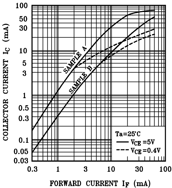
I_C - I_F
