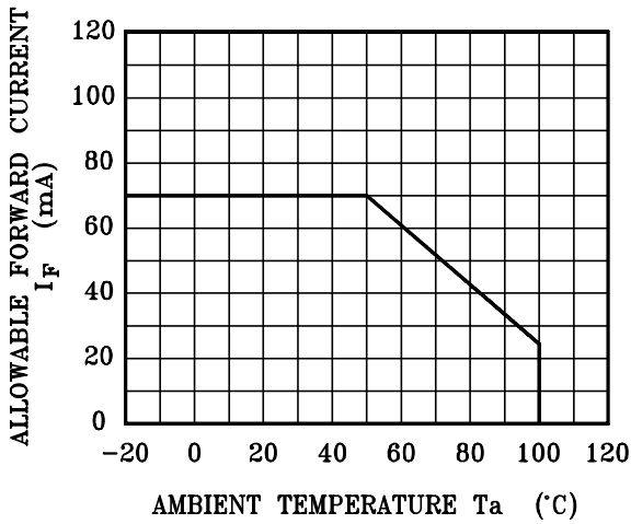
I_F - T_a
