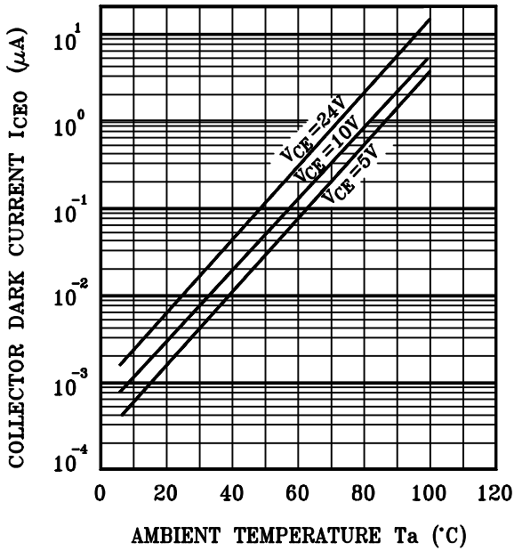
I_{CE0} - T_a
