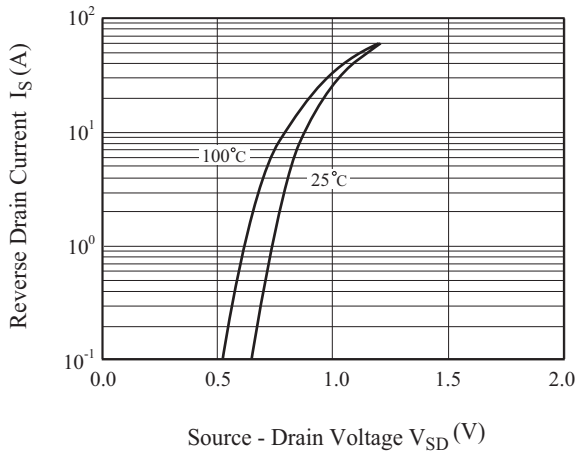
Fig7. I_S - V_{SD}
