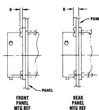
Thru-Bulkhead Receptacle
