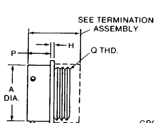
SOLDER KPT01/MS3111
