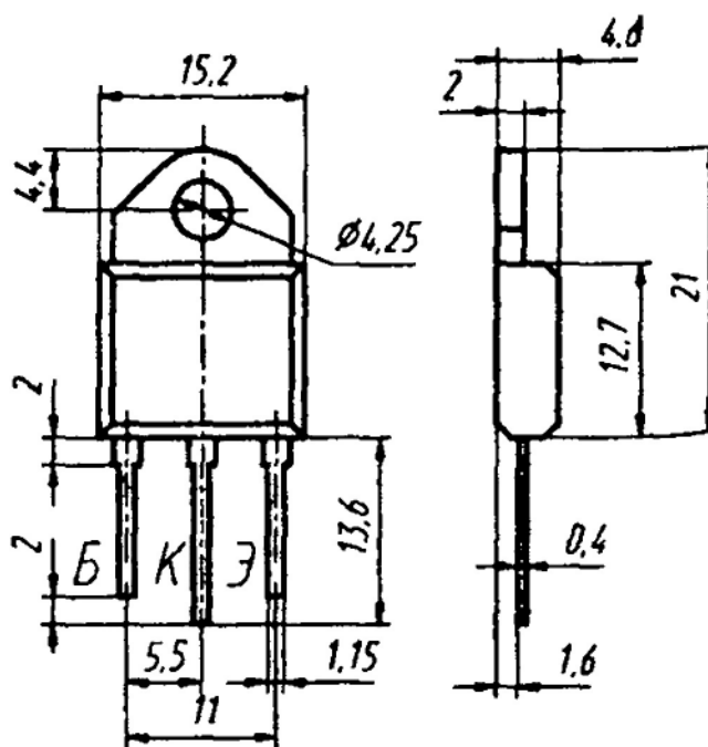
KT819(A1-Г1)
