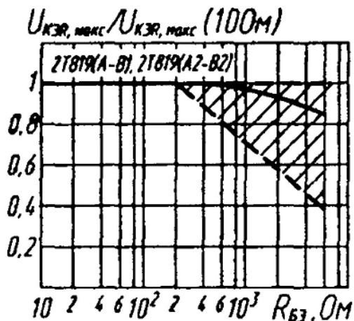
Зона возможных положений зависимости максимально допустимого напряжения коллектор—эмиттер от сопротивления база—эмиттер
