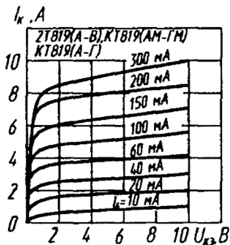
Выходные характеристики
