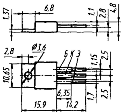
2T819(A2-B2), KT819(A-Г)
