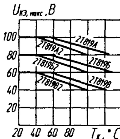
Зависимости максимально допустимого напряжения коллектор—эмиттер от температуры корпуса
