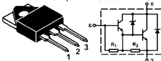
1-база 2-коллектор 3-эмиттер
