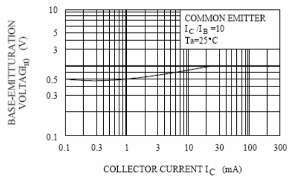
V_{BE(sat)} - I_C
