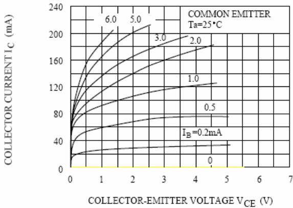
I_C - V_{CE}
