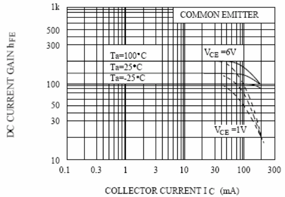
h_{FE} - I_C
