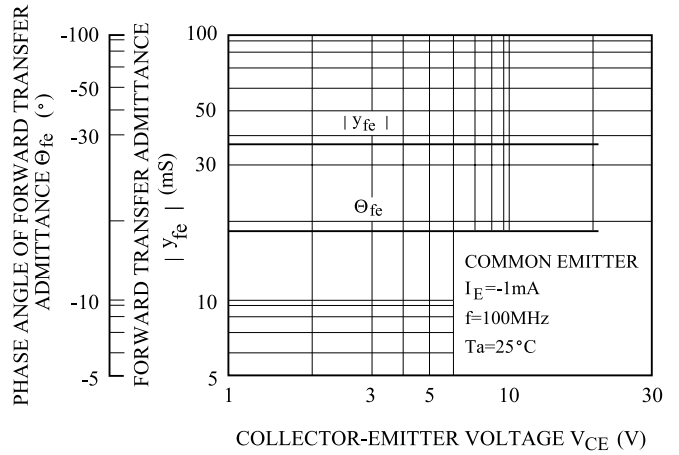
|y_{fe}|, \Theta_{fe} - V_{CE}
