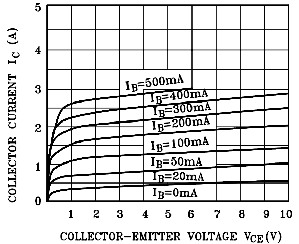
I_C - V_{CE}
