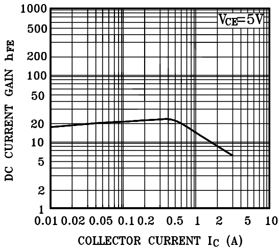
h_{FE} - I_C
