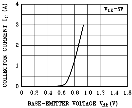
I_C - V_{BE}
