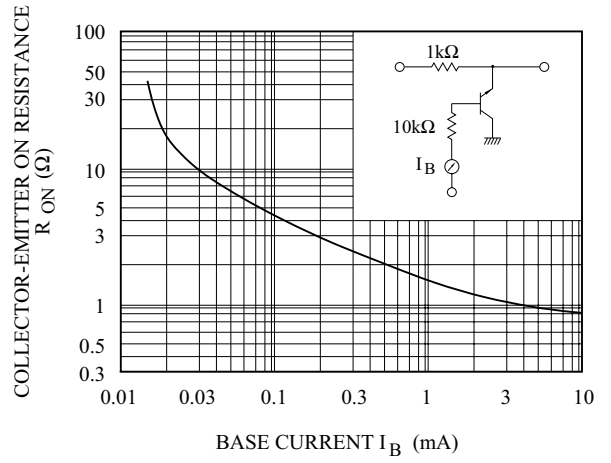
R_{ON} - I_B
