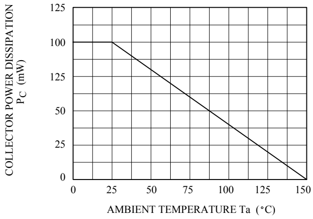
P_c - T_a
