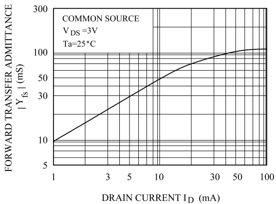
|Y_{fs}| - I_D
