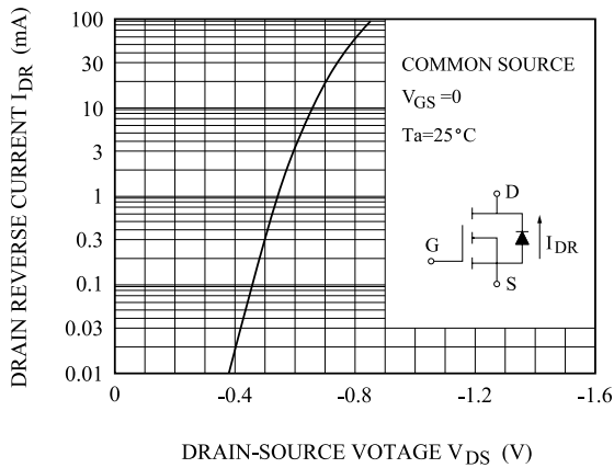
I_{DR} - V_{DS}
