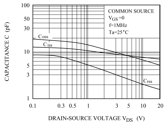
C - V_{DS}
