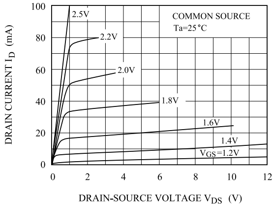
I_D - V_{DS}
