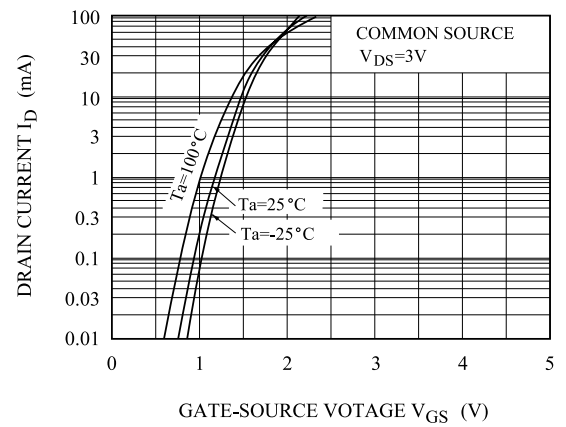
I_D - V_{GS}
