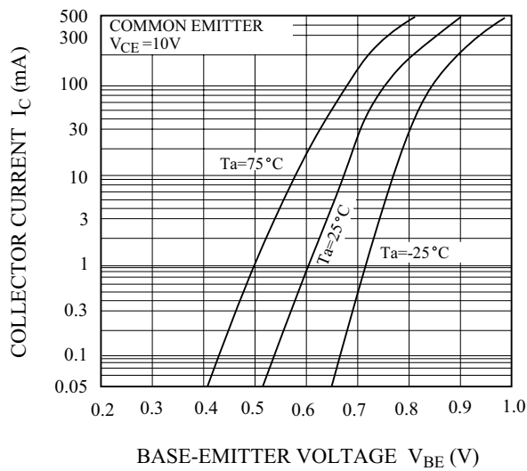
I_C - V_{BE}
