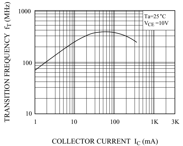
f_T - I_C
