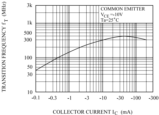
f_T - I_C
