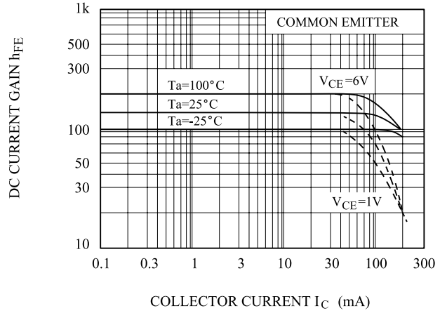
h_{FE} - I_C
