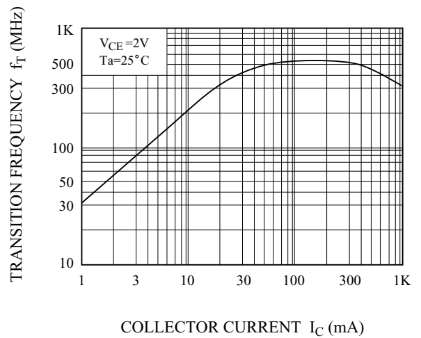
f_T - I_C
