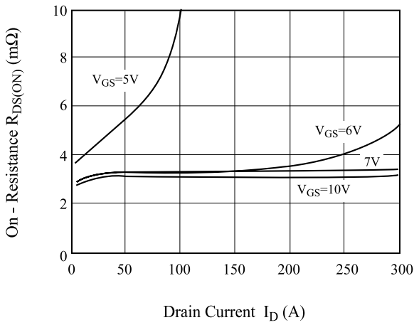
Fig7. R_{DS(ON)} - I_D
