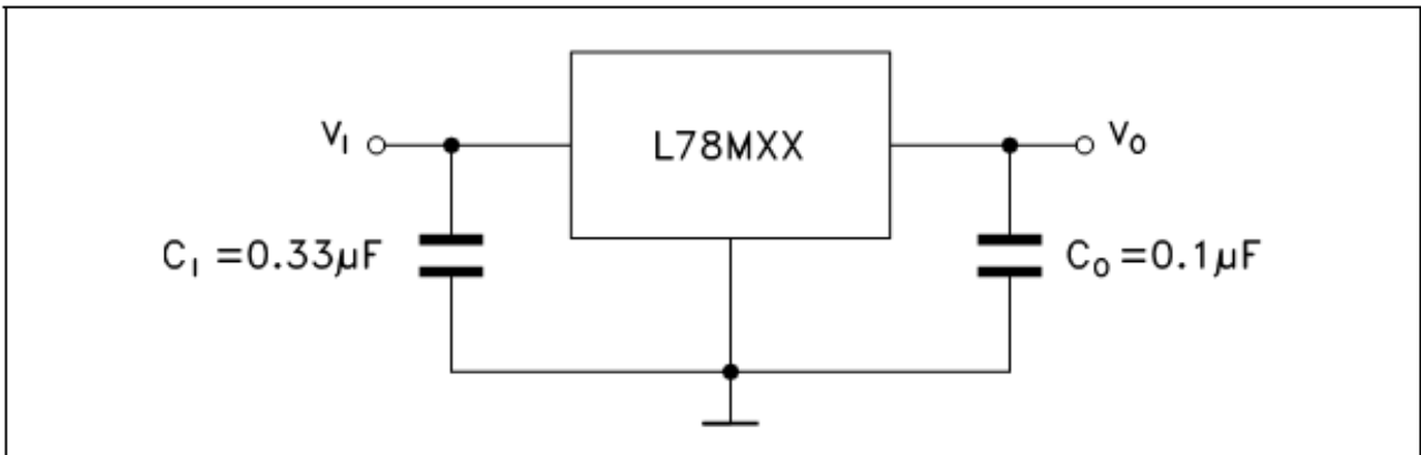
Figure 5. DC parameter
