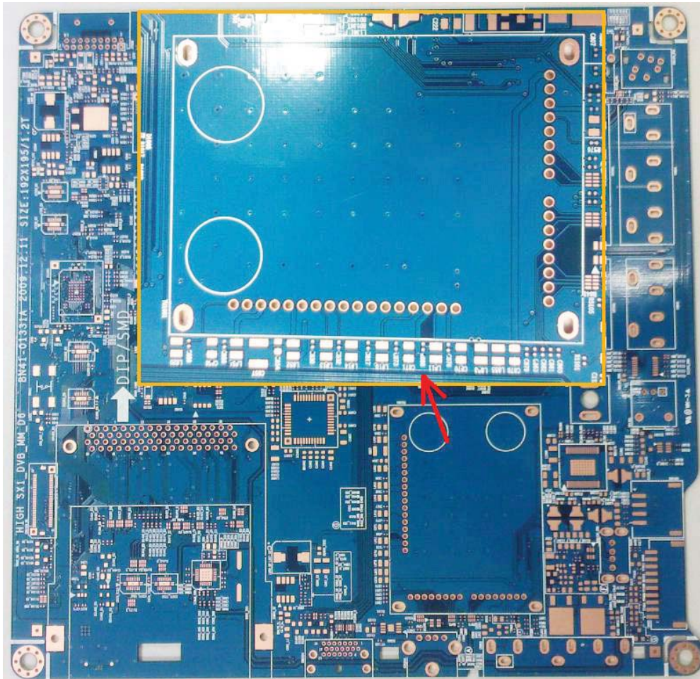
MAINBOARD(B)
