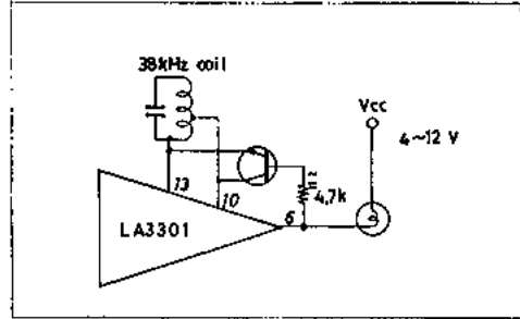
第33図 モノ・ステレオ自動切換えの改良
