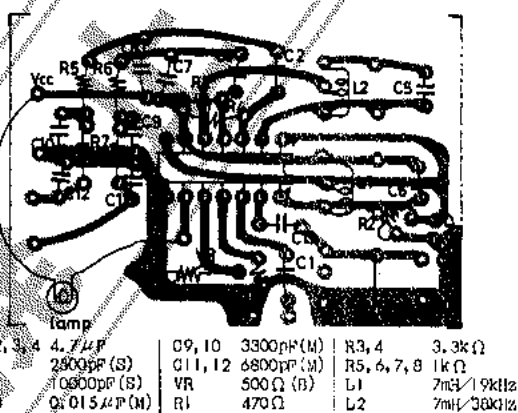
第12図 プリントパターン例(銅箔面)
