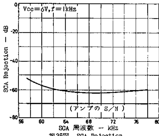
第35図 SCA Rejection
