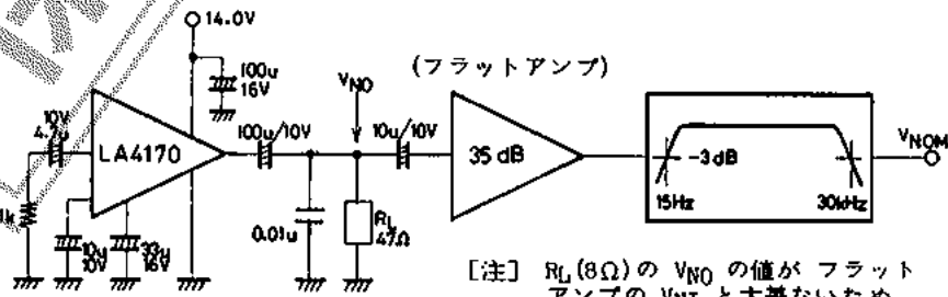
測定回路 3 (ch 1 を示す) V_{NO}
