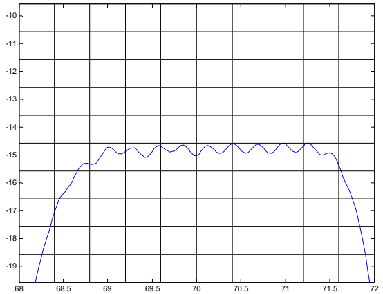
Phase Linearity( f_0 \pm 1.5\text{MHz} )
