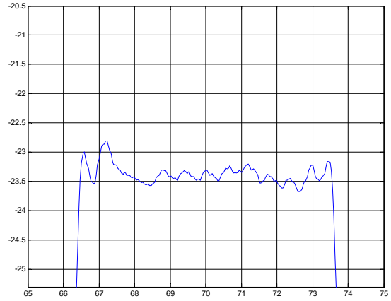
Phase Linearity( f_0 \pm 3.4\text{MHz} )
