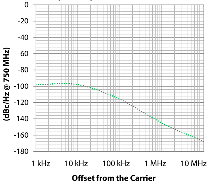
Phase Noise (dBc/Hz)
