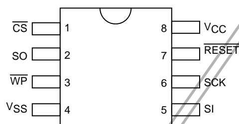
図 1 : ピン配置図
