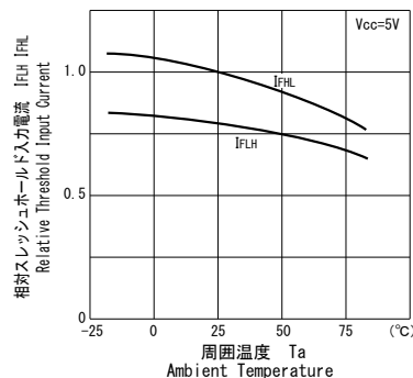
■ 相対スレッシュホールド入力電流/ 周囲温度特性 I_{FLH}, I_{FHL}/T_a
