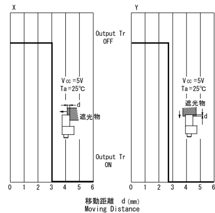
■位置検出特性
