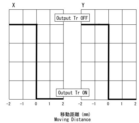
*1 位置検出特性図
