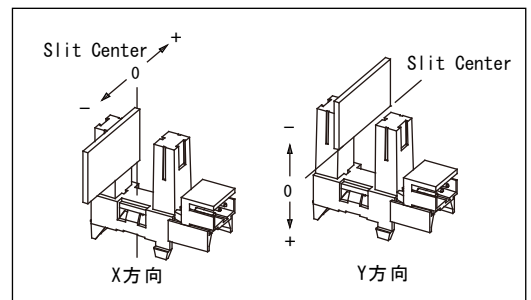
*1 位置検出特性図
