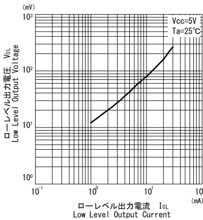
■ ローレベル出力電圧/ ローレベル出力電流特性 V_{OL}/I_{OL}
