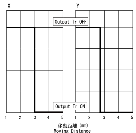
*1 位置検出特性測定方法
