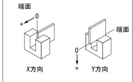
*1 位置検出特性測定方法
