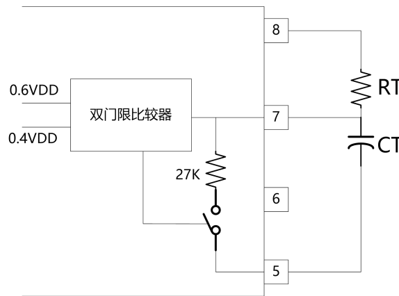
图3 振荡器内部工作原理
