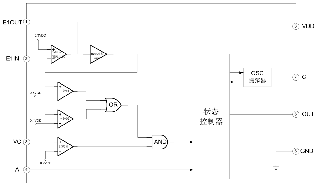
图2 功能框图
