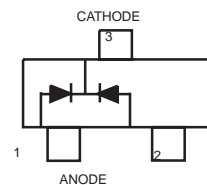
SC-70
