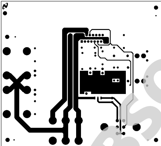
Top Layer
