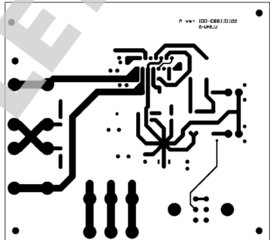
Bottom Layer
