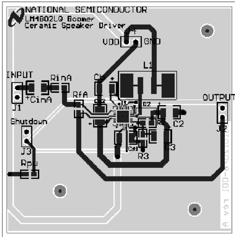
Composite Layer
