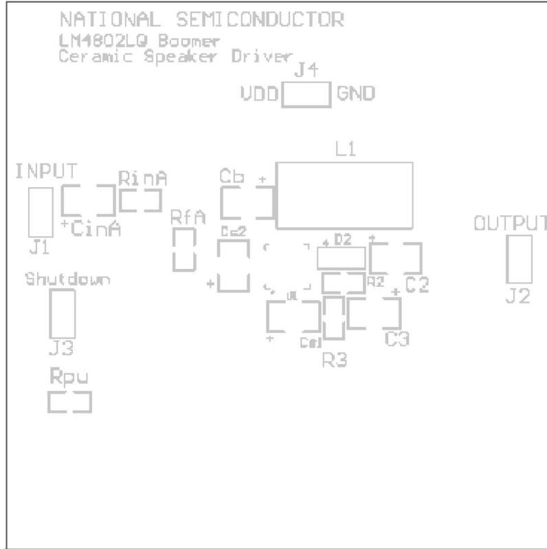
Top Overlay
