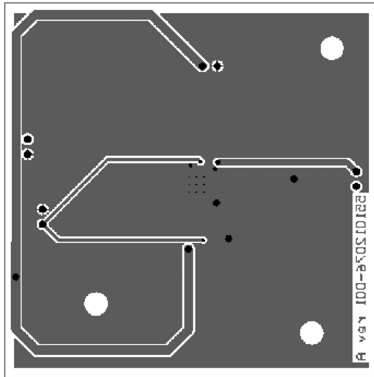
Bottom Layer
