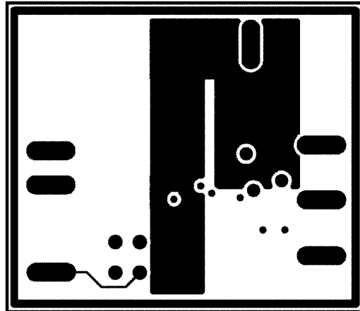
FIGURE 12. Layer 3 (V DD )
