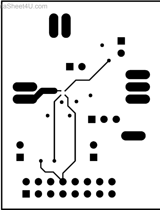
Bottom Layer
