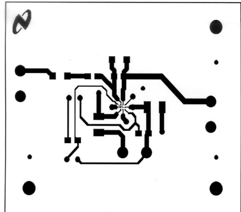
Top Layer
