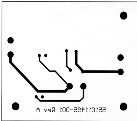
Bottom Layer
