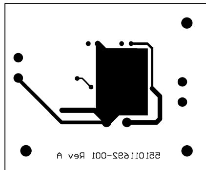
Bottom Layer
