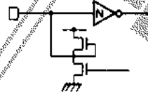
入出力共通ハイスレッシュヨルド入力オープンドレイン 出力 (H, PU)
