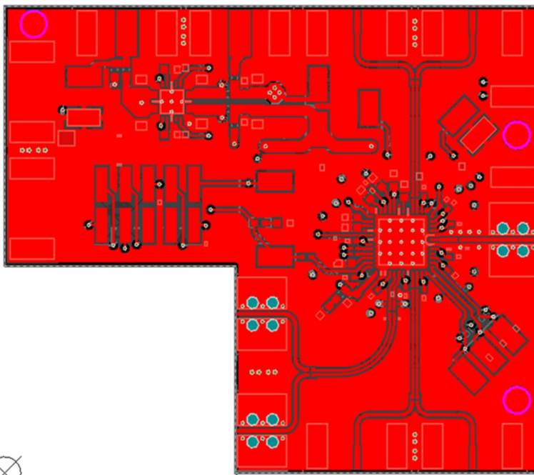
Figure 94. Top Layer
