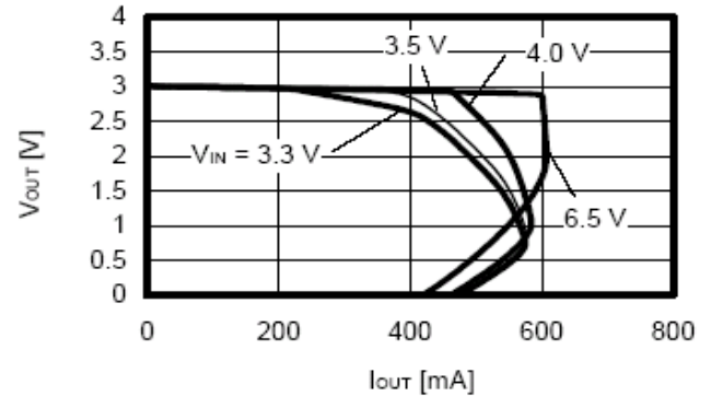
LN1130 (3.0V)
