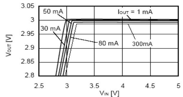
LN1130 (3.0V)
