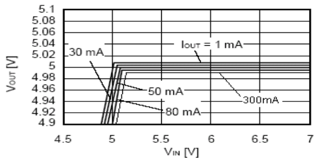
LN1130 (5.0V)
