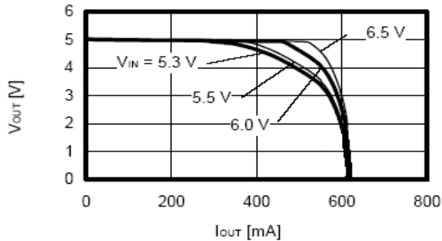
LN1130 (5.0V)
