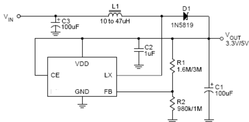
电路 1 LN2267 在便携式仪器中的典型应用
