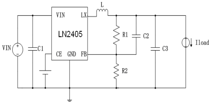
Circuit3
