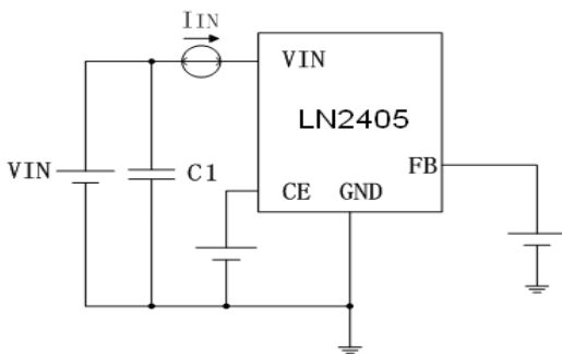
Circuit3
