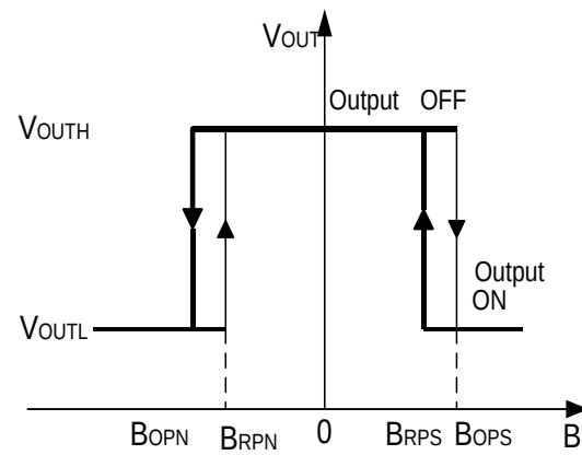
输出开关特性曲线
