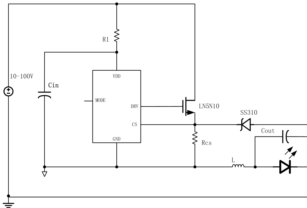
LN2552MR 浮地模式应用
