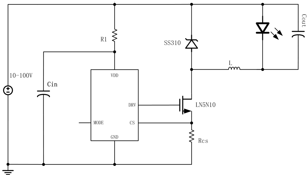
LN2552MR 共地模式应用
