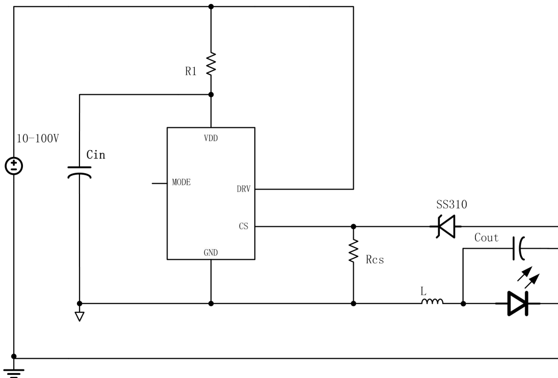
LN2552SR 浮地模式应用
