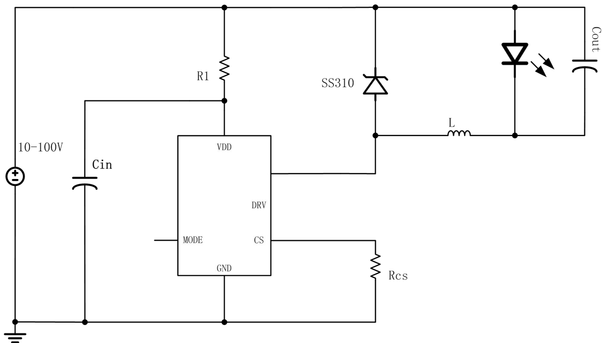
LN2552SR 共地模式应用
