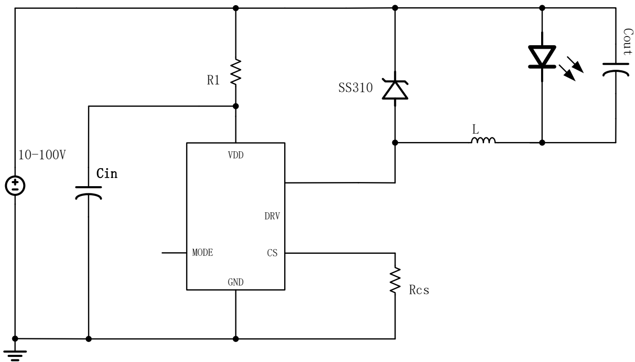
LN2557SR 共地模式应用
