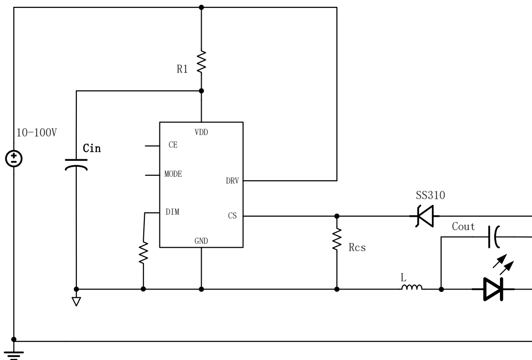
LN2558SR 浮地模式应用
