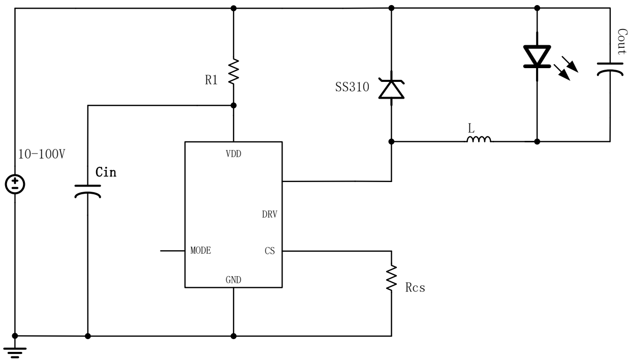
LN2558SR 共地模式应用
