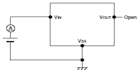
电路 2
